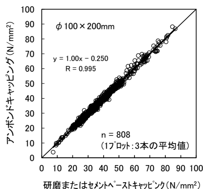
研磨またはセメントペーストキャッピング供試体とアンボンドキャッピング供試体の強度との関係 ※φ125×200mm についても同様の結果が得られております
